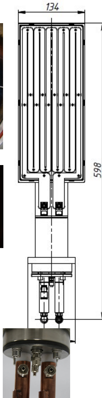
Heater 400 ЛЦМК.232.00.00.00.000
